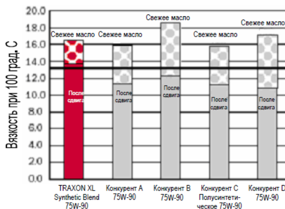
Сравнительный анализ вязкостей свежего масла и после испытания на сдвиг KRL при 1000С, GL-5 75W-90
